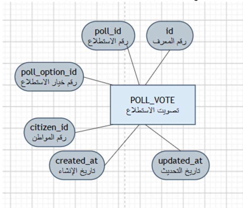
الشكل (38.4) يبين كينونة تصويت الاستطلاع
