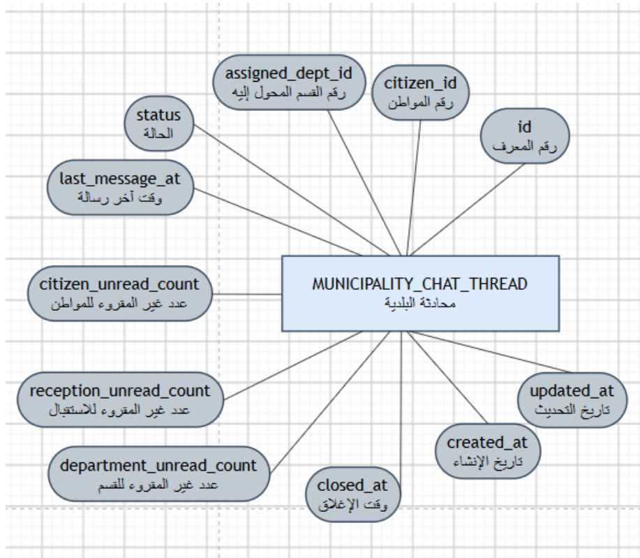
الشكل (40.4) يبين كينونة محادثة البلدية
