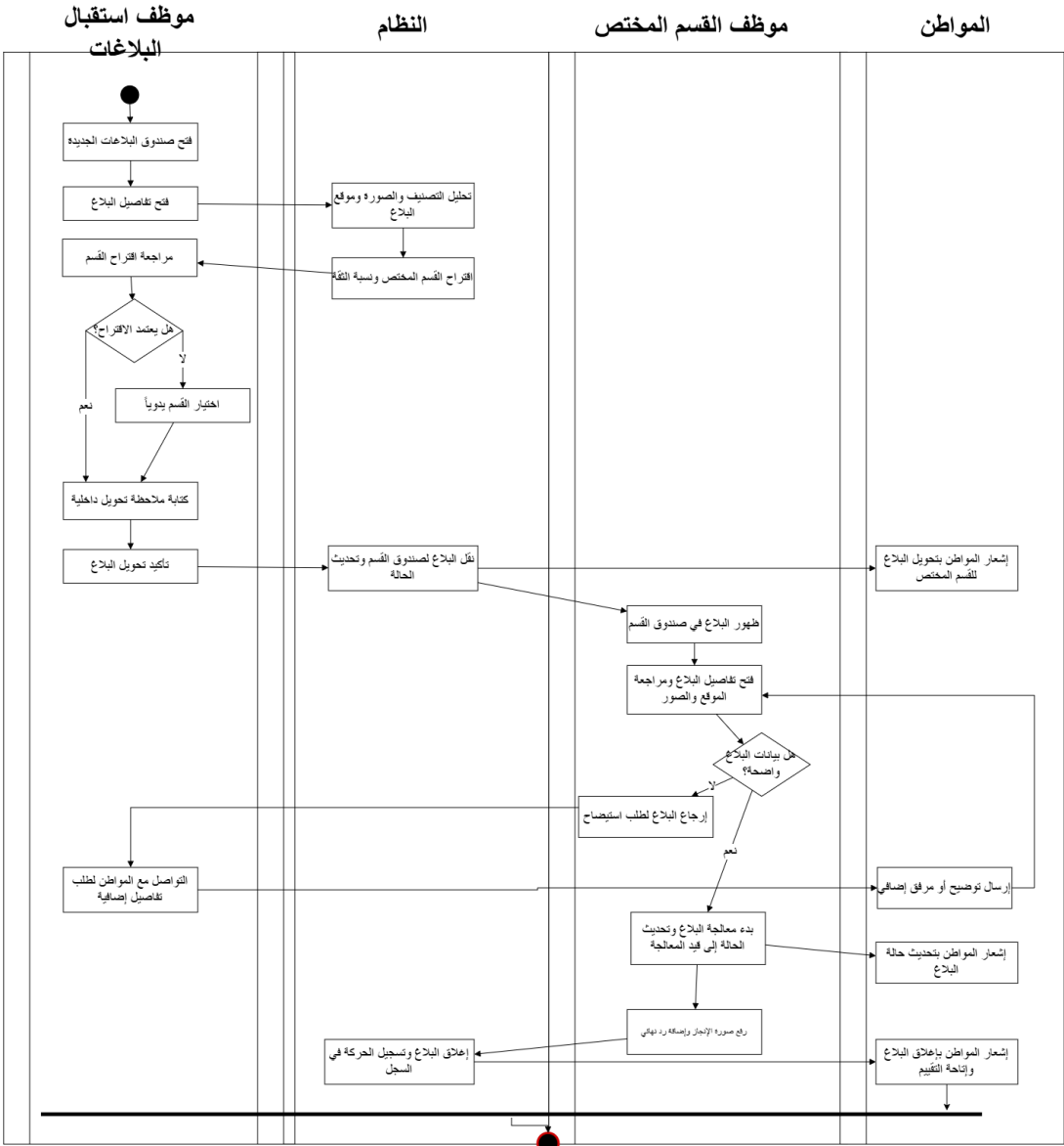
شكل (3.4) يوضح مخطط نشاط لعملية تحويل البلاغ إلى القسم المختص ومعالجته.
