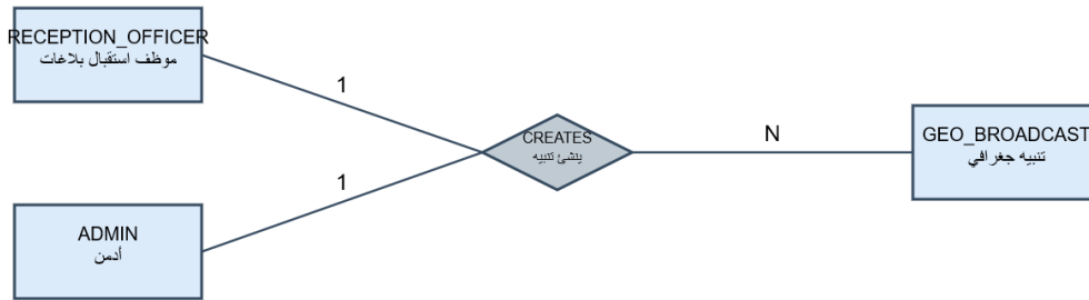
الشكل (77.4) يبين العلاقة بين موظف استقبال بلاغات و أدمن و تنبيه جغرافي
