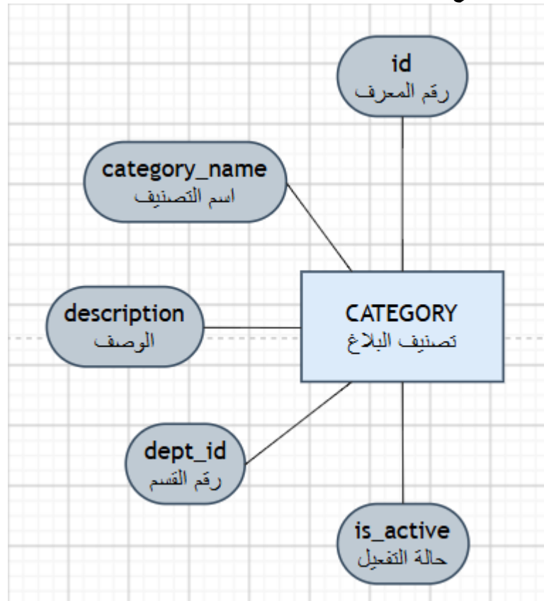
الشكل (10.4) يبين كينونة تصنيف البلاغ
