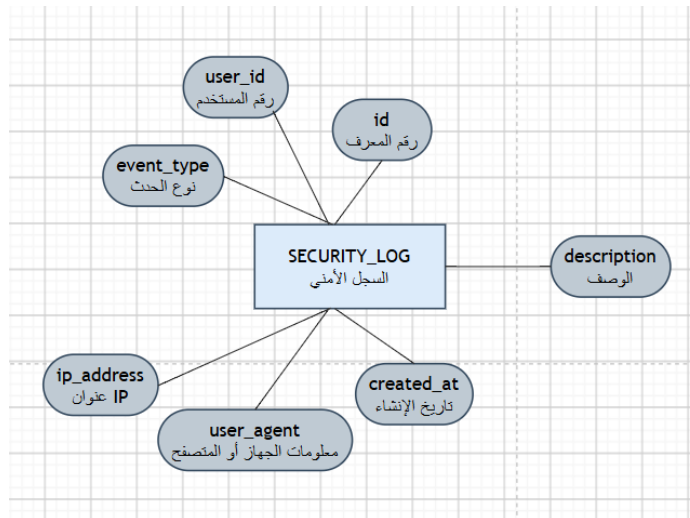
الشكل (24.4) يبين جدول السجل الامني
