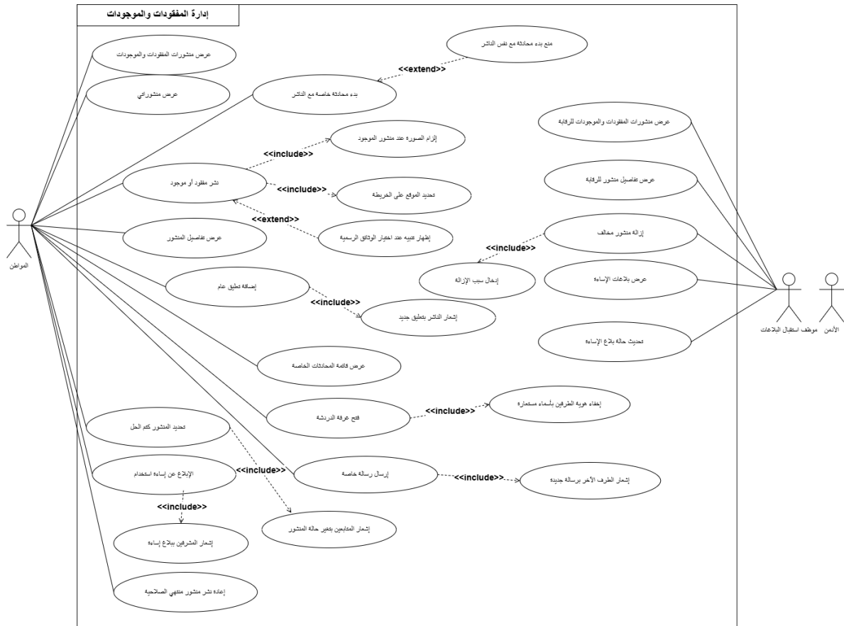
الشكل 16.3 يبين حالات استخدام إدارة المفقودات والموجودات
