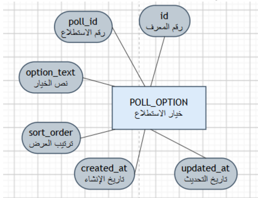
الشكل (37.4) يبين كينونة خيار استطلاع
