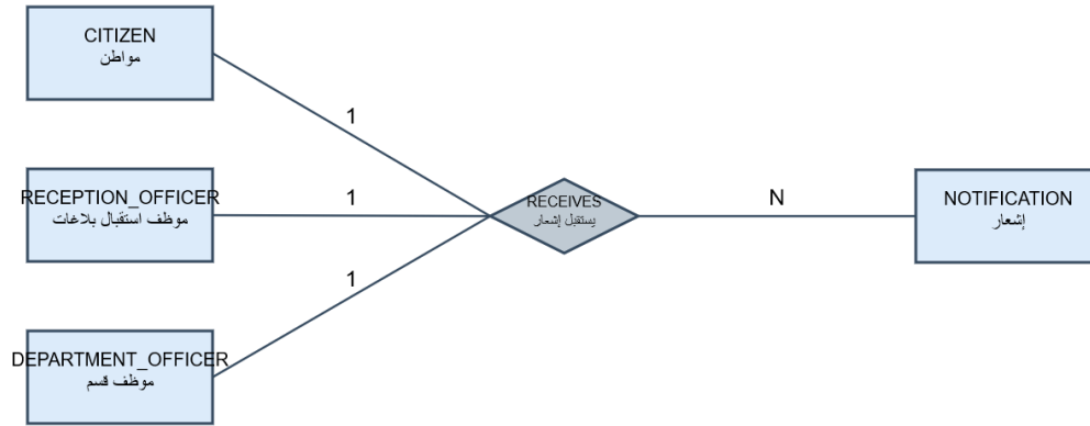
الشكل (107.4) يبين العلاقة بين مواطن و موظف استقبال بلاغات و موظف قسم و إشعار
