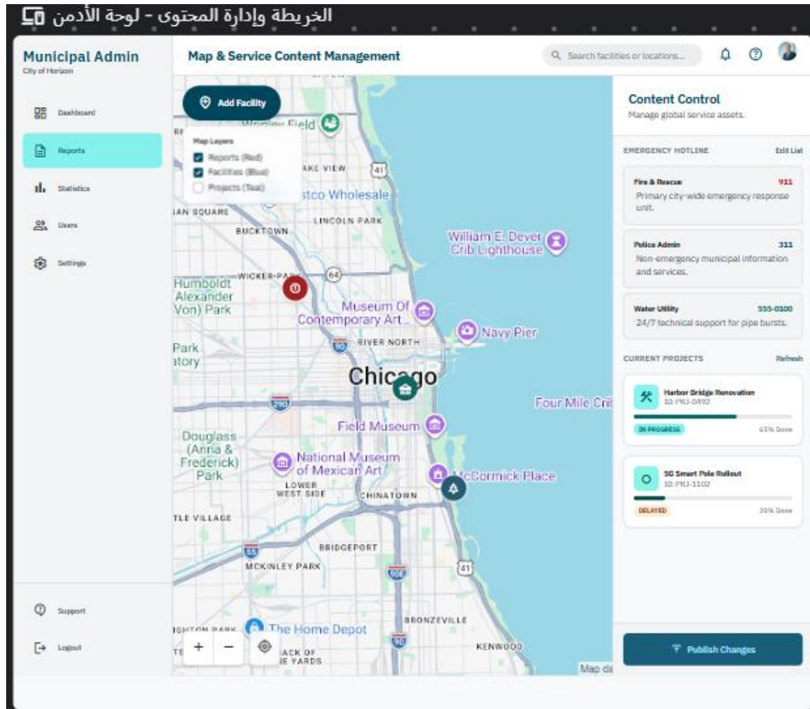
الشكل 117.4 (يوضح التصميم المبدئي لواجهة إدارة المحتوى و الخريطة للأدمن
