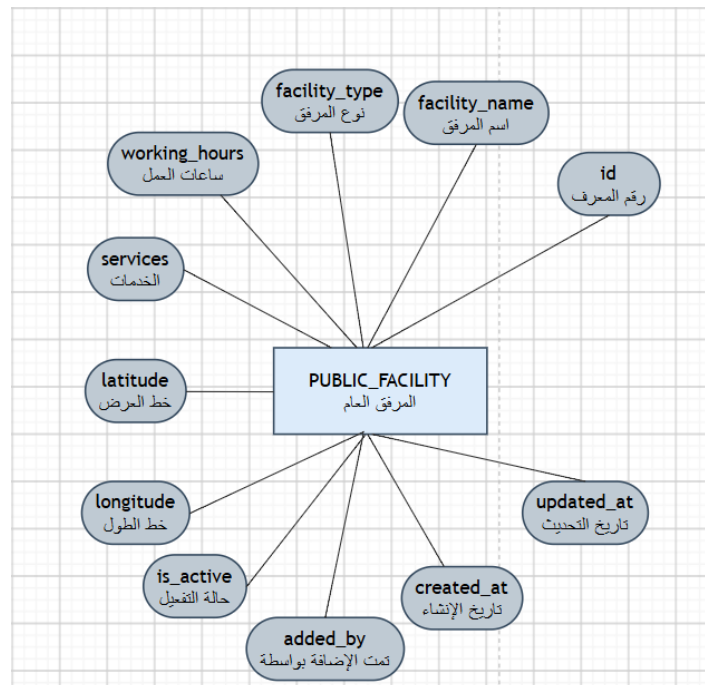
الشكل (22.4) يبين كينونة المرفق العام
