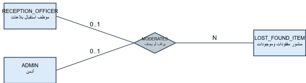
الشكل (83.4) يبين العلاقة بين موظف استقبال بلاغات و أدمن و منشور مفقودات وموجودات
