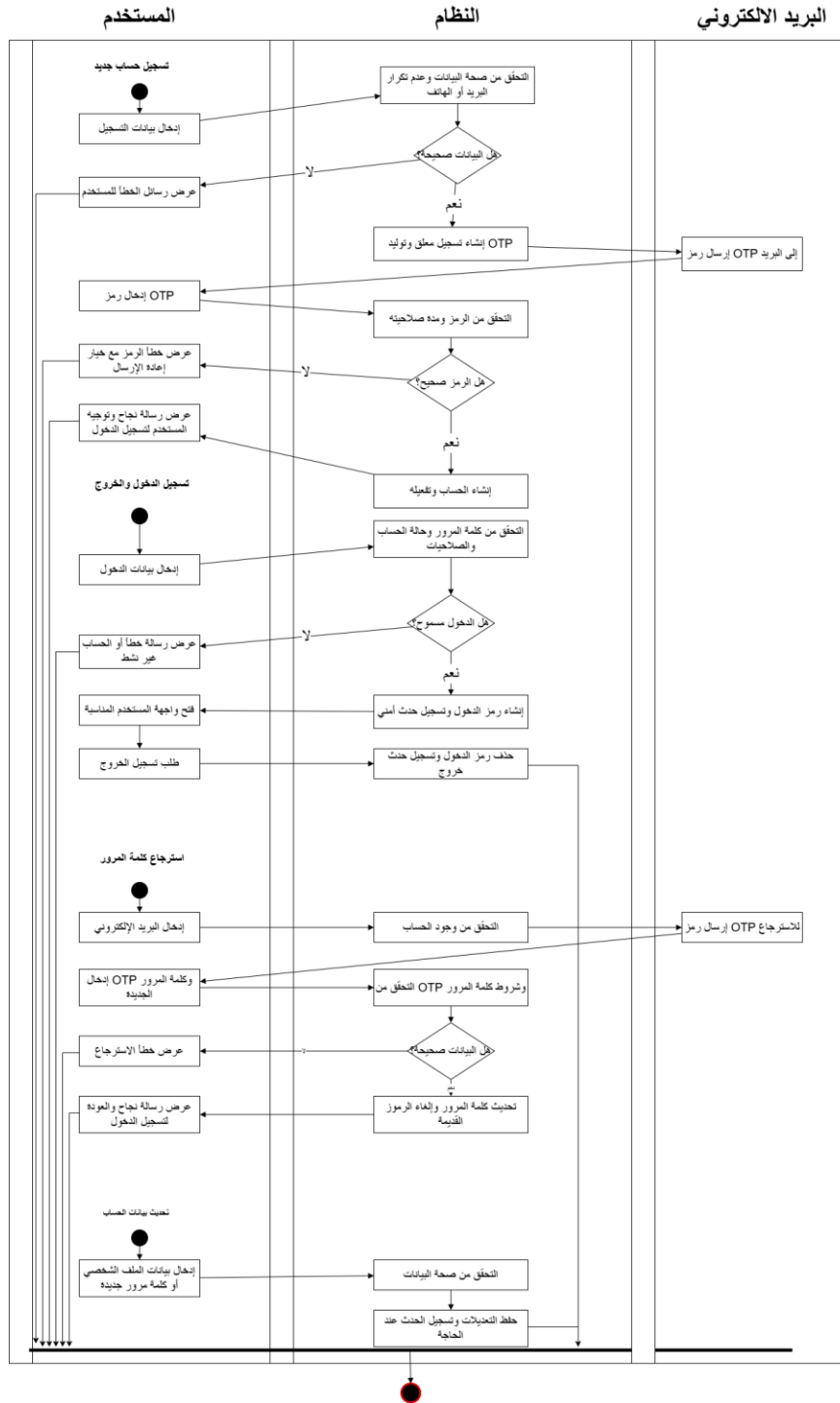
شكل (1.4) يوضح مخطط النشاط الخاص بإدارة المصادقة والحسابات
