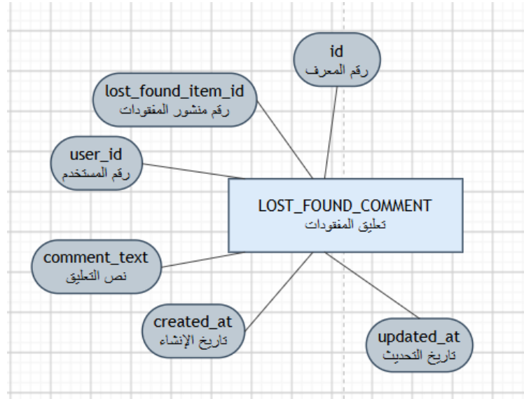
الشكل (32.4) يبين كينونة تعليق المفقودات
