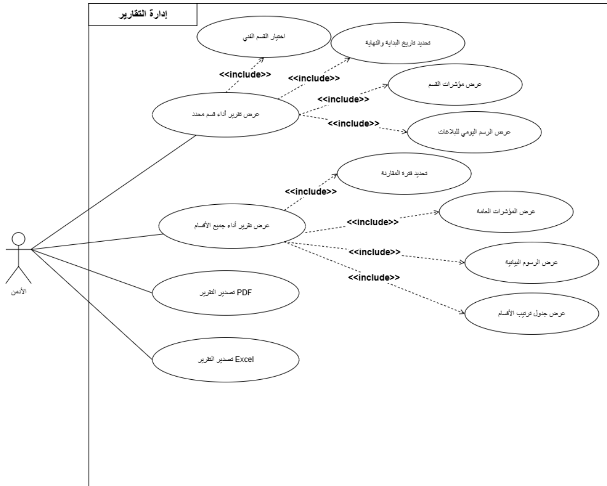
الشكل 10.3 يبين حالات استخدام إدارة التقارير
