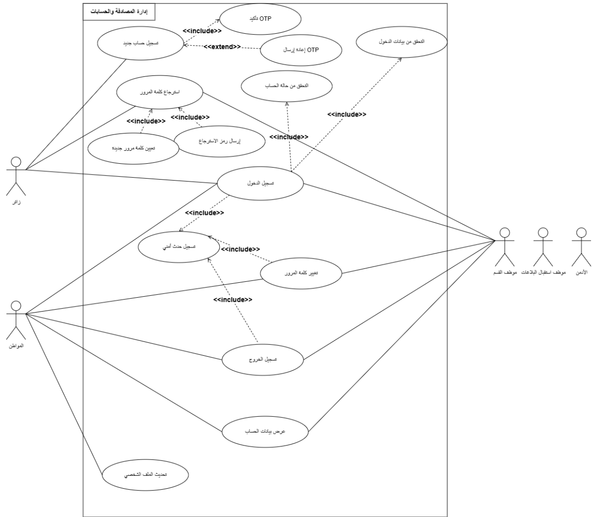
يبين حالات استخدام إدارة المصادقة و الحسابات 6.3 الشكل
