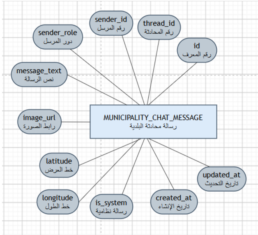
الشكل (41.4) يبين كينونة رسالة محادثة البلدية
