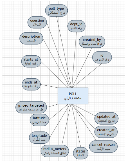
الشكل (36.4) يبين كينونة استطلاع الرأي
