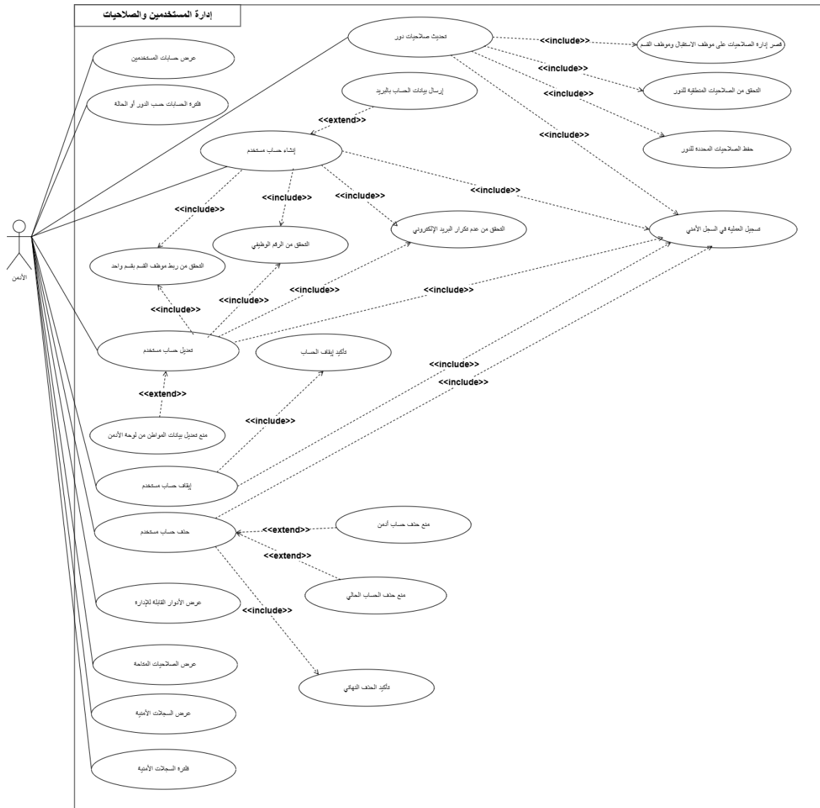
الشكل 19.3 يبين حالات استخدام إدارة المستخدمين والصلاحيات
