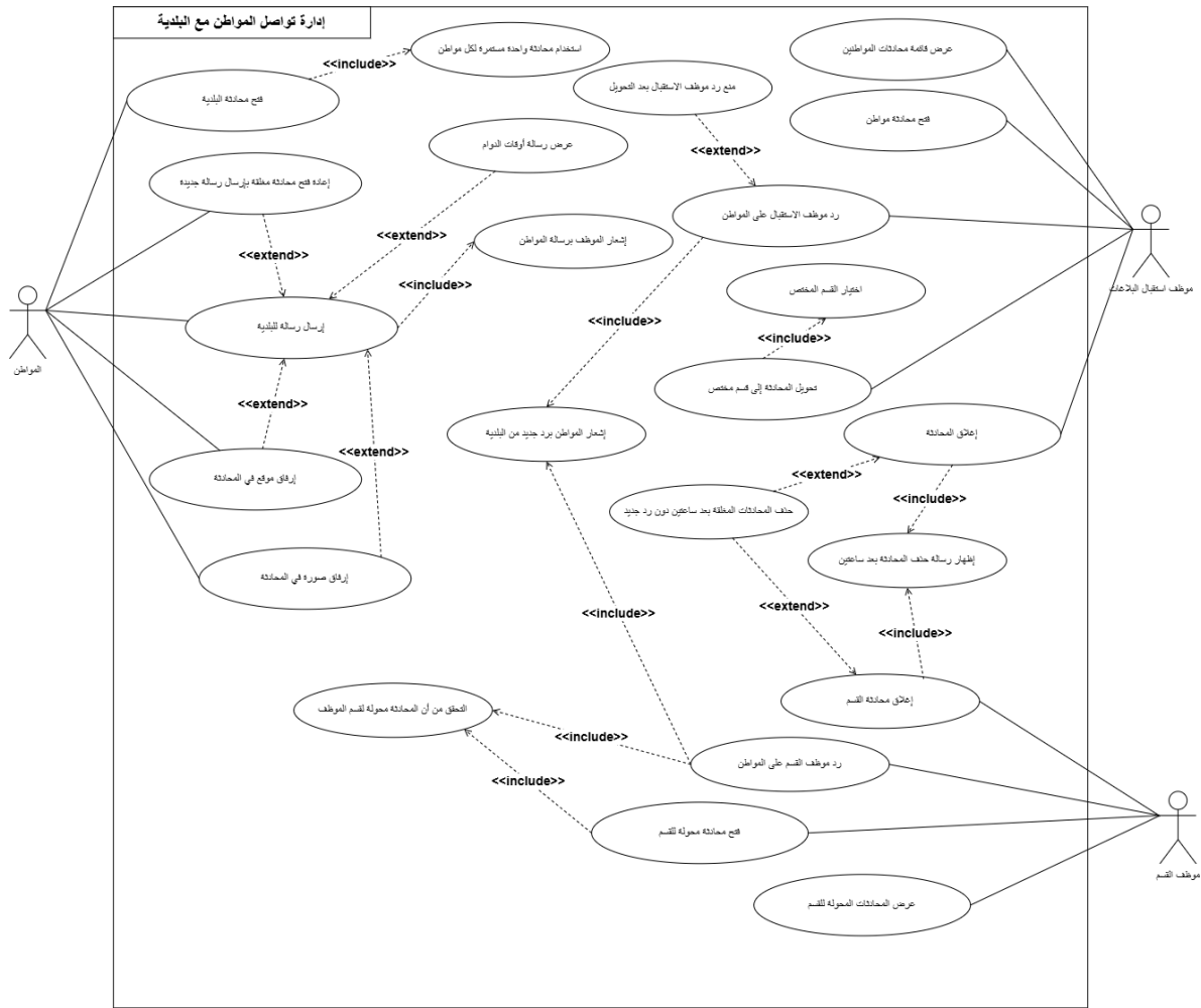
الشكل 18.3 يبين حالات استخدام إدارة تواصل المواطنين مع البلدية
