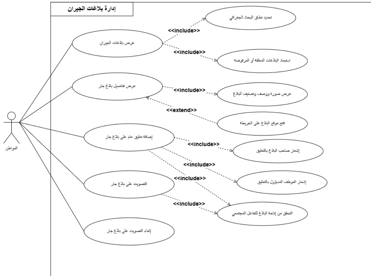
الشكل 13.3 يبين حالات استخدام إدارة بلاغات الجيران
