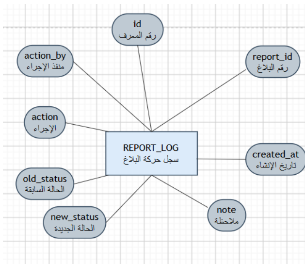
الشكل (14.4) يبين كينونة إجراء البلاغ
