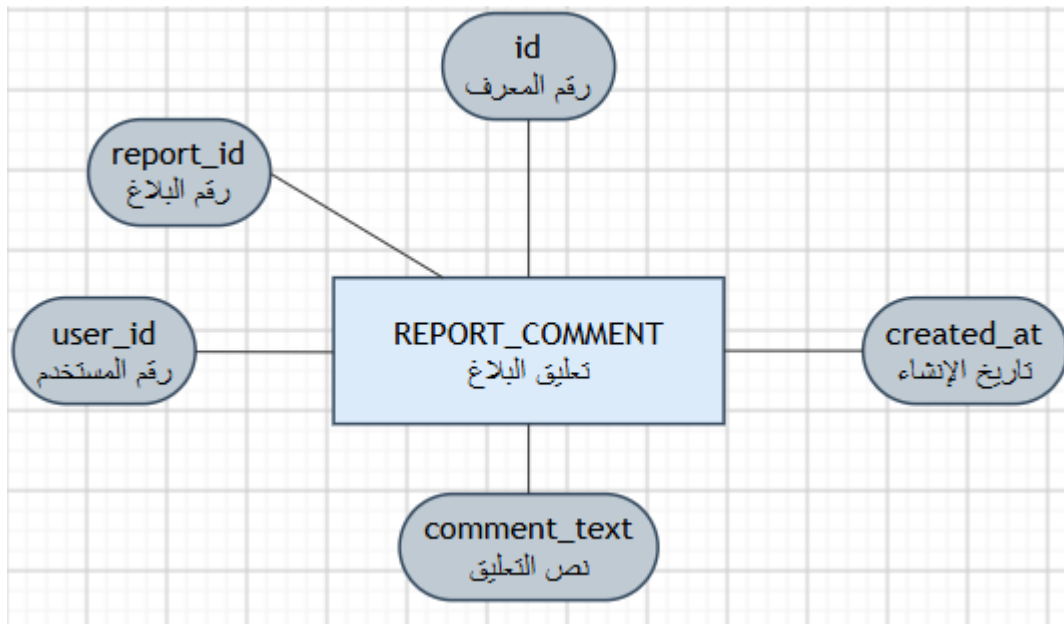
الشكل (15.4) يبين كينونة تعليق البلاغ
