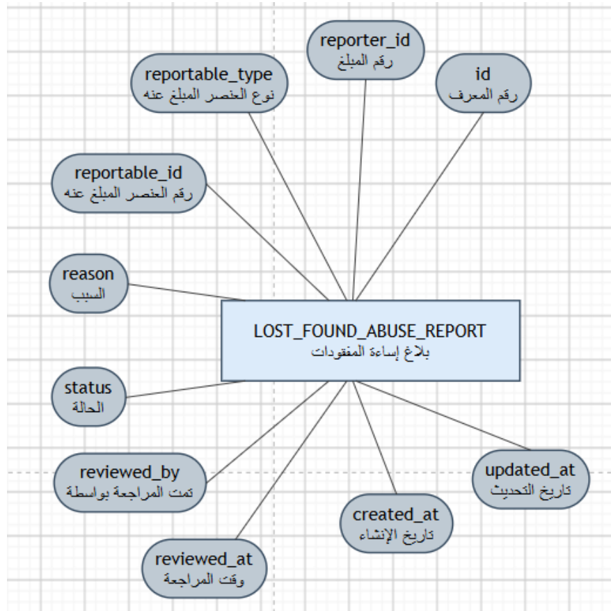
الشكل (35.4) يبين كينونة بلاغ اساءة المفقودات
