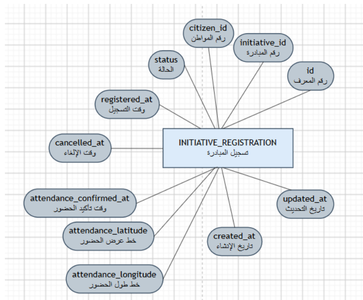
الشكل (28.4) يبين كينونة تسجيل مبادرة
