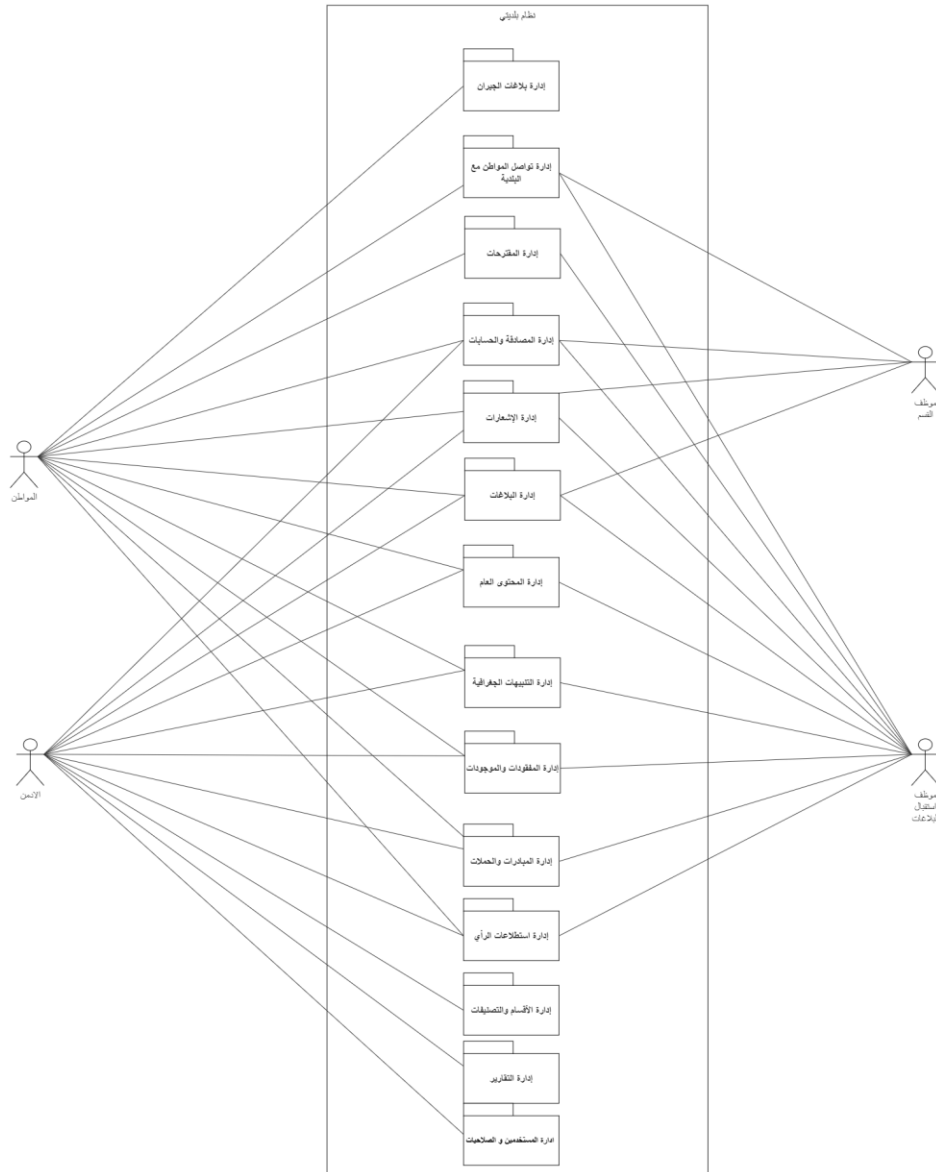
الشكل 5.3: مخطط حالة الاستخدام لنظام بلدي
