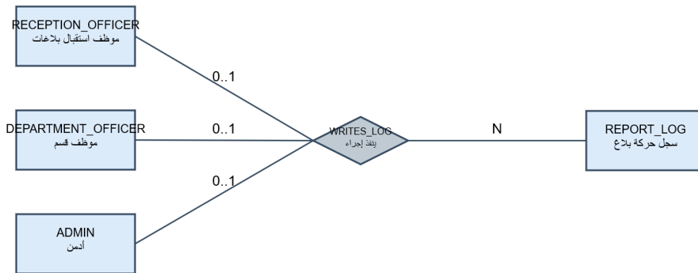
الشكل 57.4 (يبين العلاقة بين موظف استقبال بلاغات و موظف قسم و أدمن و سجل حركة بلاغ)
