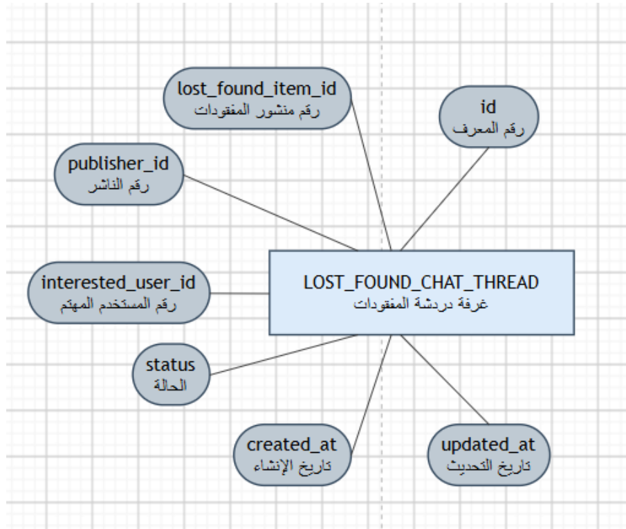
الشكل (33.4) يبين كينونة غرفة دردشة المفقودات
