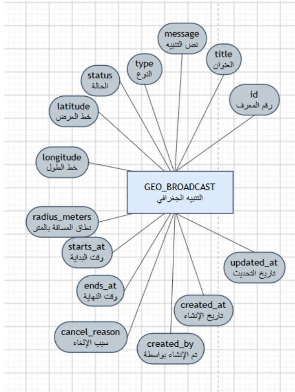
الشكل (29.4) يبين كينونة التنبيه الجغرافي
