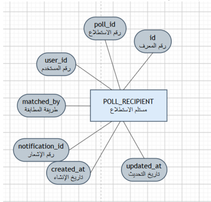
الشكل (39.4) يبين كينونة مستلم الاستطلاع
