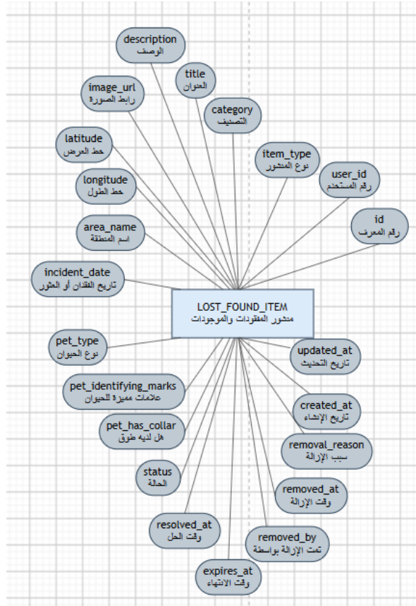
الشكل (31.4) يبين كينونة منشور مفقودات و الموجودات
