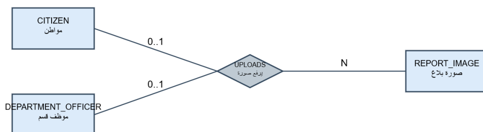
الشكل (55.4) يبين العلاقة بين مواطن و موظف قسم و صورة
