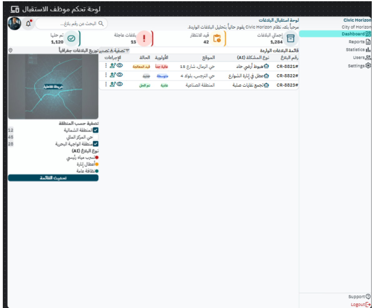
الشكل (113.4) يوضح التصميم المبدئي للوحة استقبال البلاغات لموظف البلاغات
