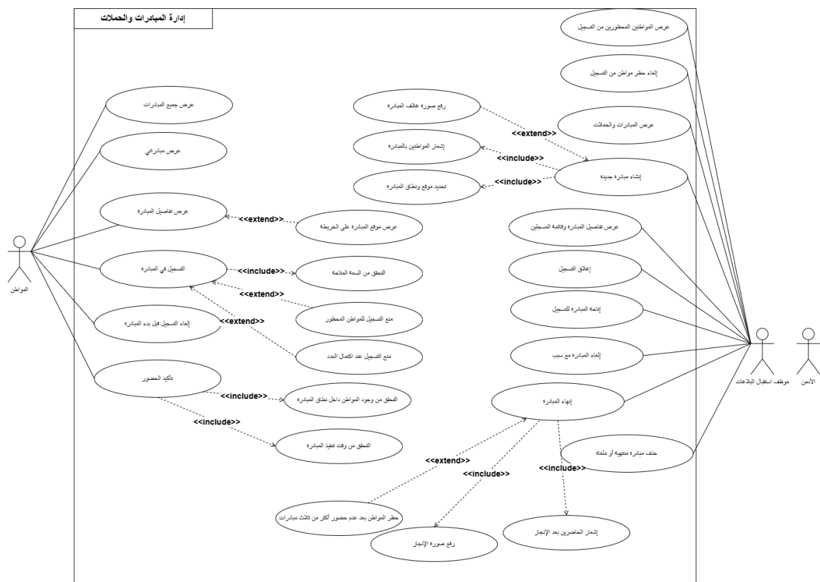
الشكل 14.3 يبين حالات استخدام إدارة المبادرات و الحملات
