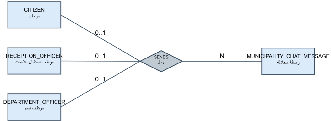
الشكل (105.4) يبين العلاقة بين مواطن و موظف استقبال بلاغات و موظف قسم و رسالة محادثة
