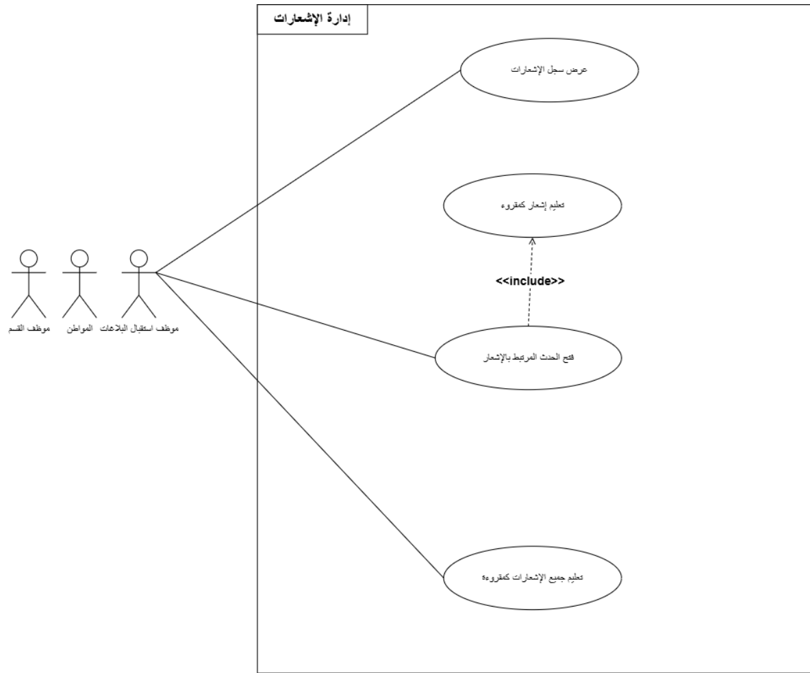
الشكل 7.3 يبين حالات استخدام ادارة الاشعارات
