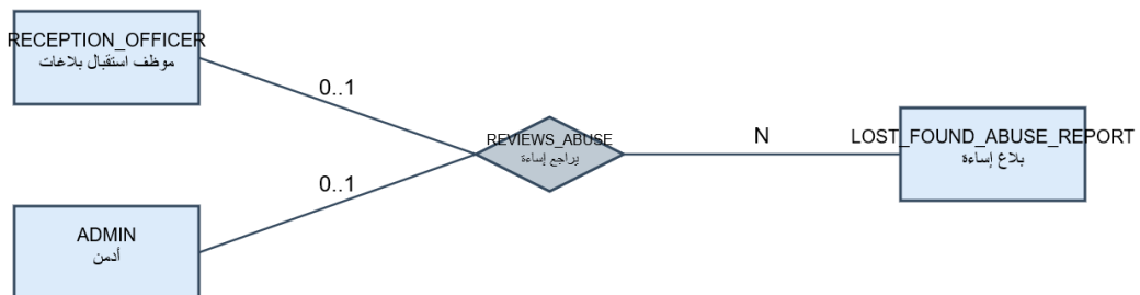
الشكل (92.4) يبين العلاقة بين موظف استقبال بلاغات و أدمن و بلاغ إساءة
