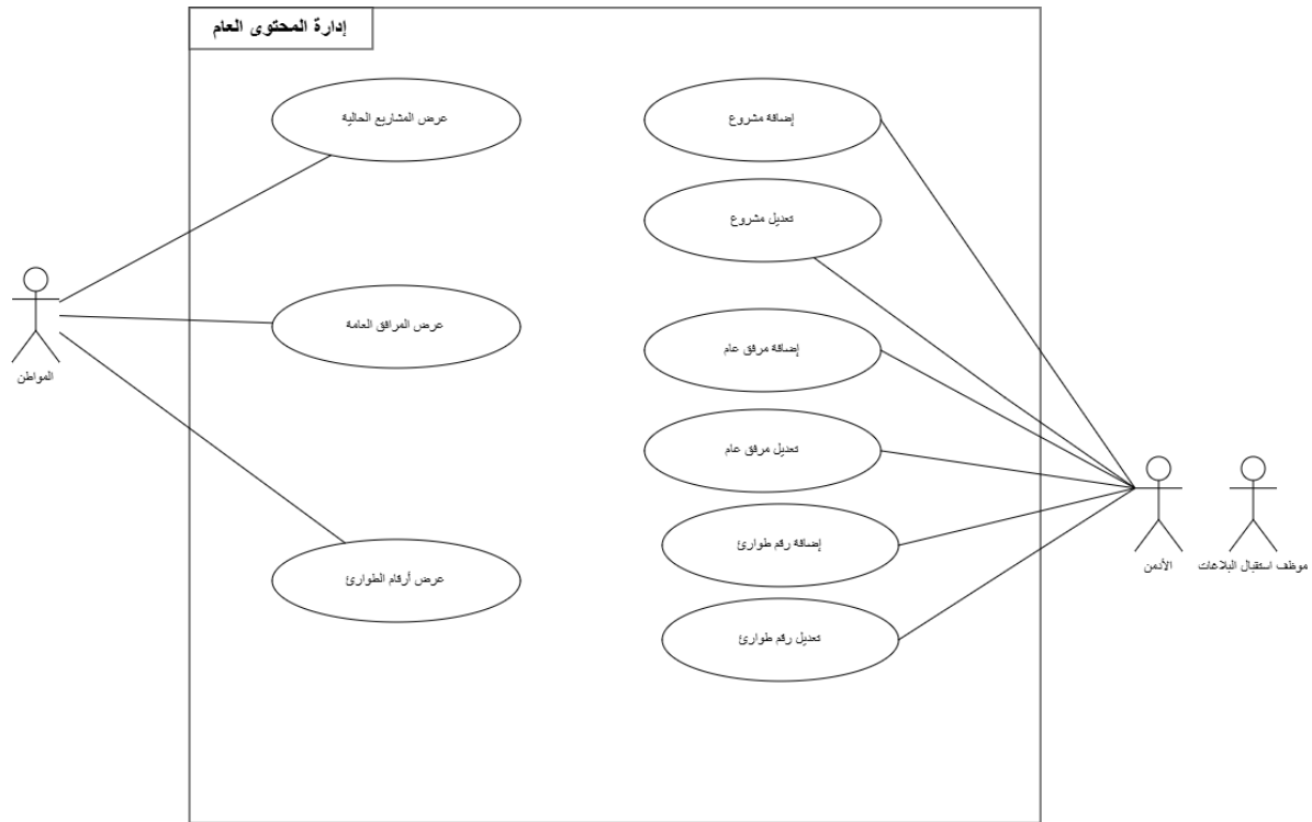
الشكل 8.3 يبين حالات استخدام إدارة المحتوى العام
