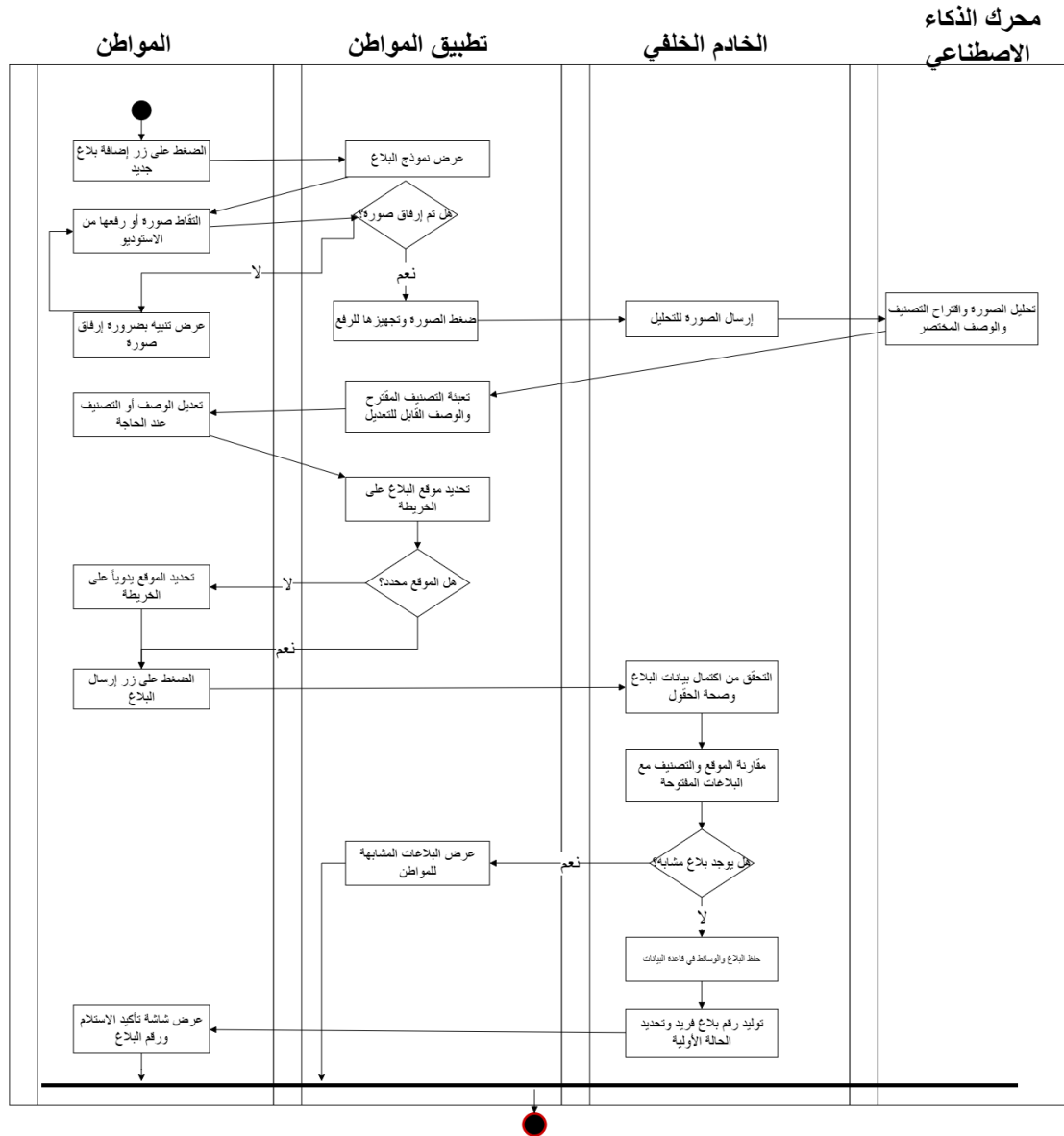
شكل (2.4) يوضح مخطط النشاط لعملية إنشاء بلاغ خدمي
