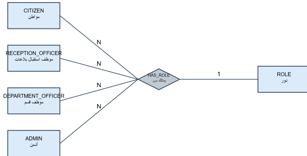
الشكل (46.4) يبين العلاقة بين مواطن و موظف استقبال بلاغات و موظف قسم و أدمن ودور
